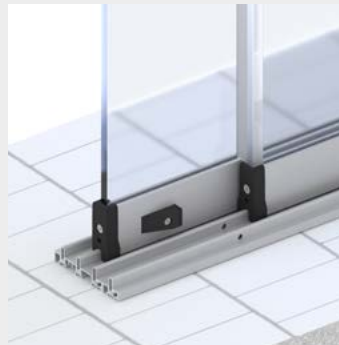
Drenaje marco inferior
