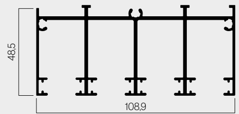
Guía superior 4 carriles Cortina de Cristal 070056
